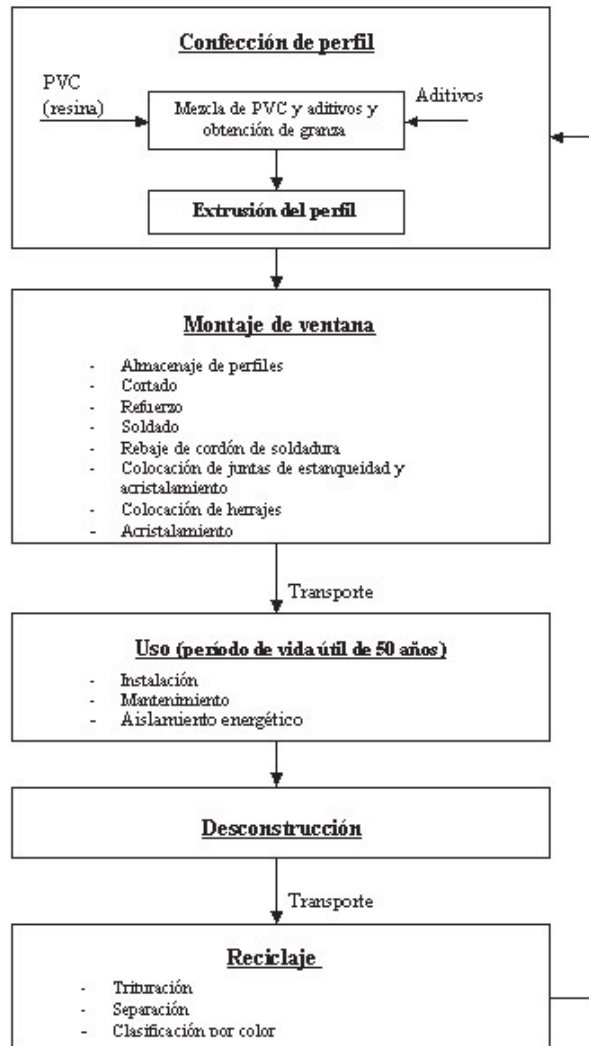
Figura 3.2: Etapas de confección y uso de perfil de PVC para ventanas
