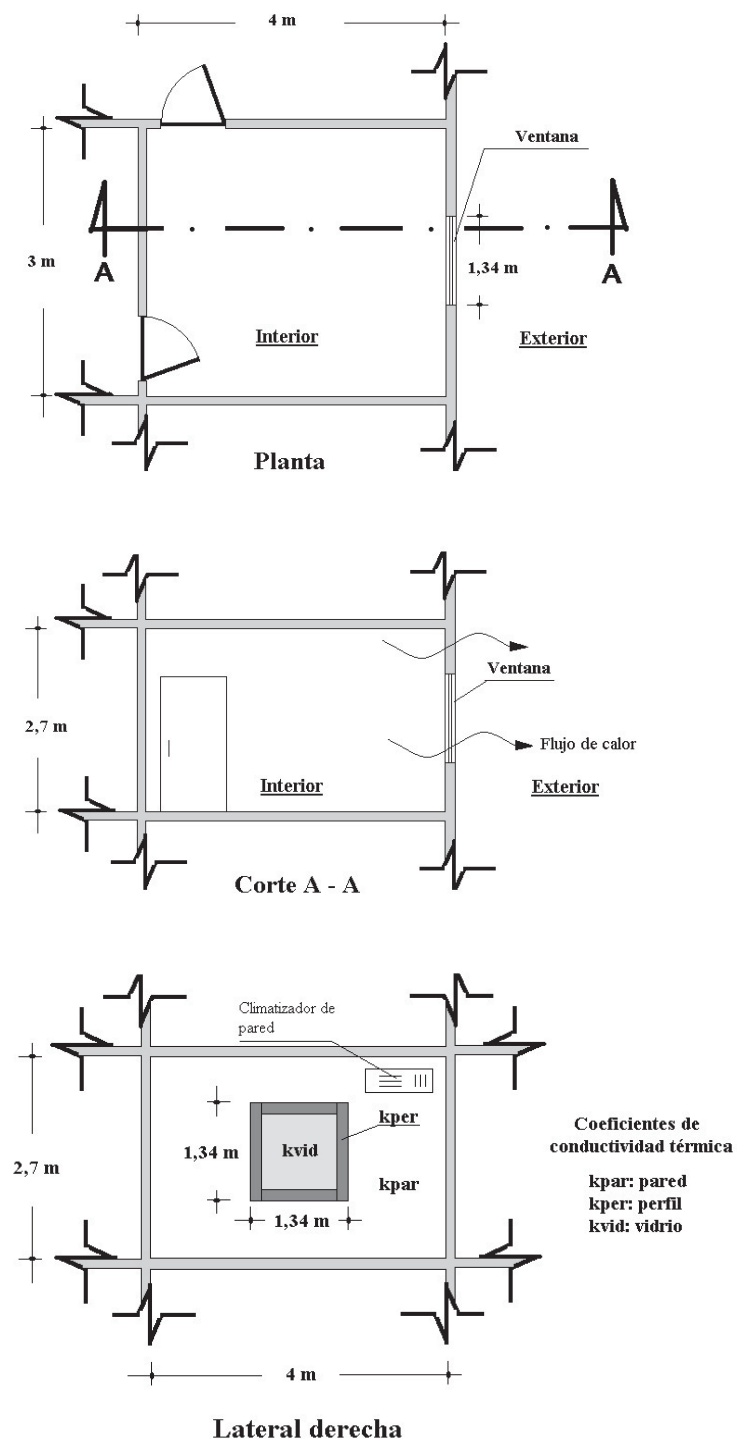
Figura 4.1: Dimensiones de la habitación de análisis
